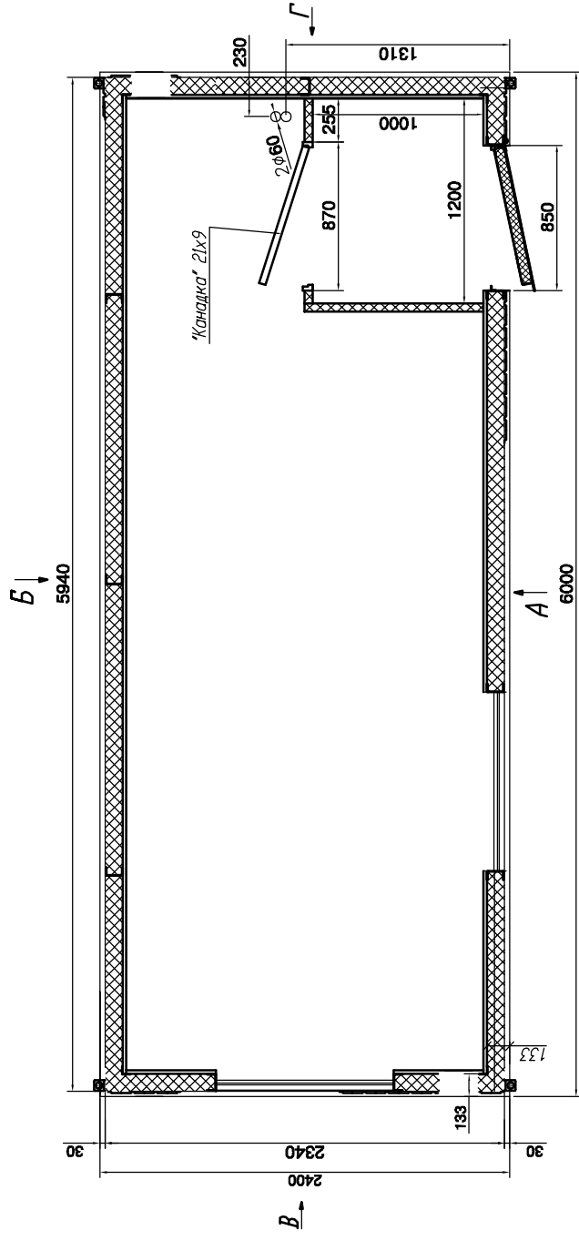
План модуля 6000x2400x2400мм
